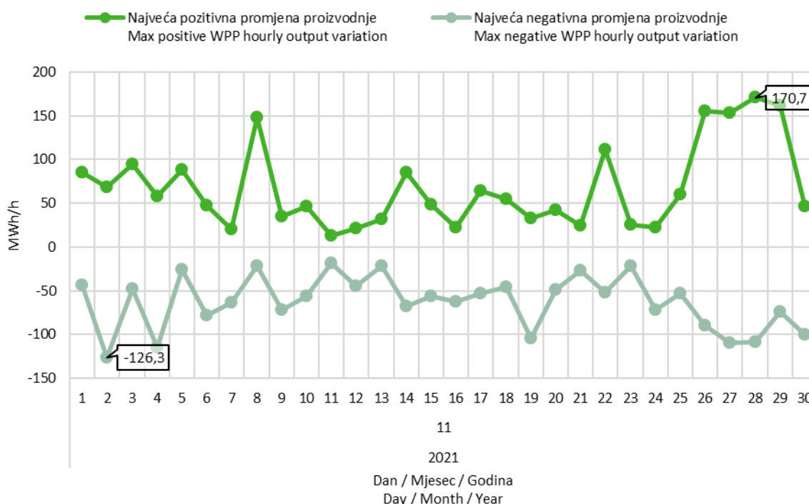
Slika 9 Maksimalna pozitivna i maksimalna negativna promjena satne proizvodnje VE u studenom 2021. godine
