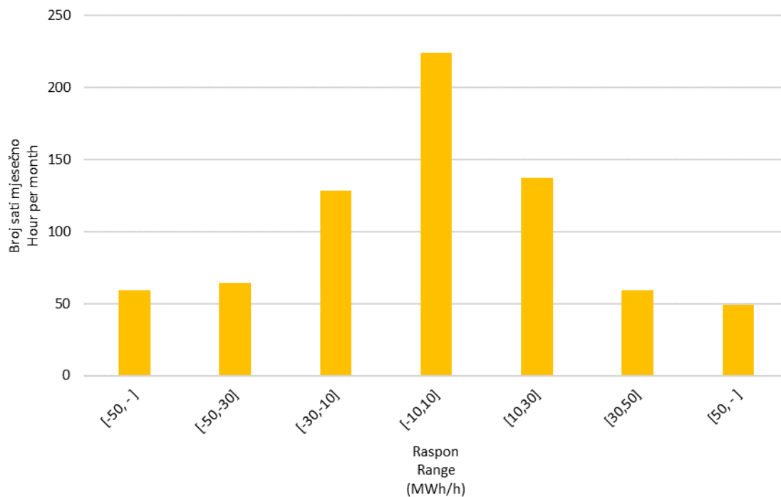
Slika 10 Statistička raspodjela satnih promjena proizvodnje VE u studenom 2021. godine
