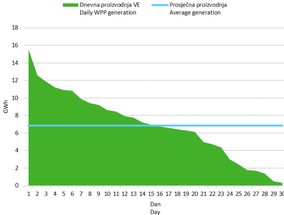
Slika 6 Krivulja trajanja dnevne proizvodnje vjetroelektrana u studenom 2021. godine
