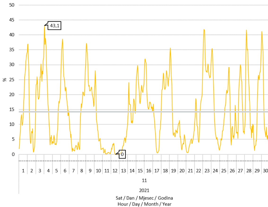
Slika 8 Udio proizvodnje vjetroelektrana u pokrivanju satnog opterećenja elektroenergetskog sustava u studenom 2021. godine
