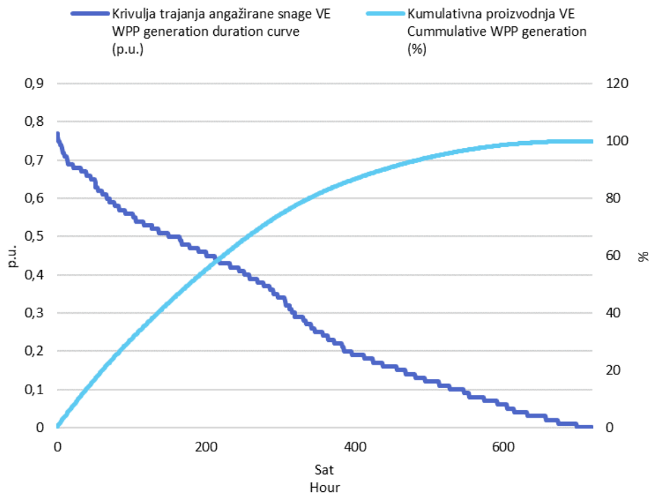
Slika 3 Krivulja trajanja angažirane snage svih VE i kumulativna proizvodnja VE u studenom 2021. godine u jediničnim vrijednostima
