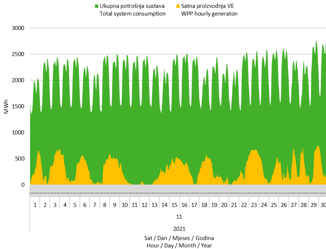
Slika 7 Usporedba satnog dijagrama opterećenja sustava i proizvodnje vjetroelektrana u studenom 2021. godine
