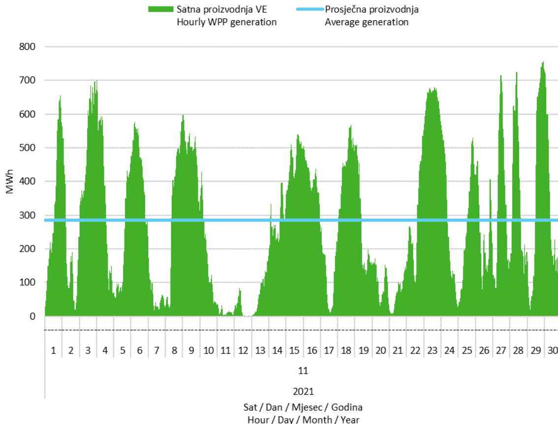
Slika 2 Satna proizvodnja svih vjetroelektrana u studenom 2021. godine
