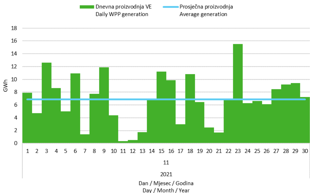
Slika 5 Dnevna proizvodnja svih vjetroelektrana u studenom 2021. godine Figure 5 Daily generation of all wind power plants in November 2021
